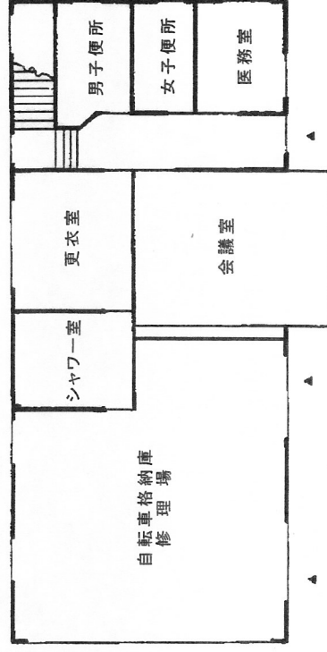
1階平面図 (214.24㎡)
